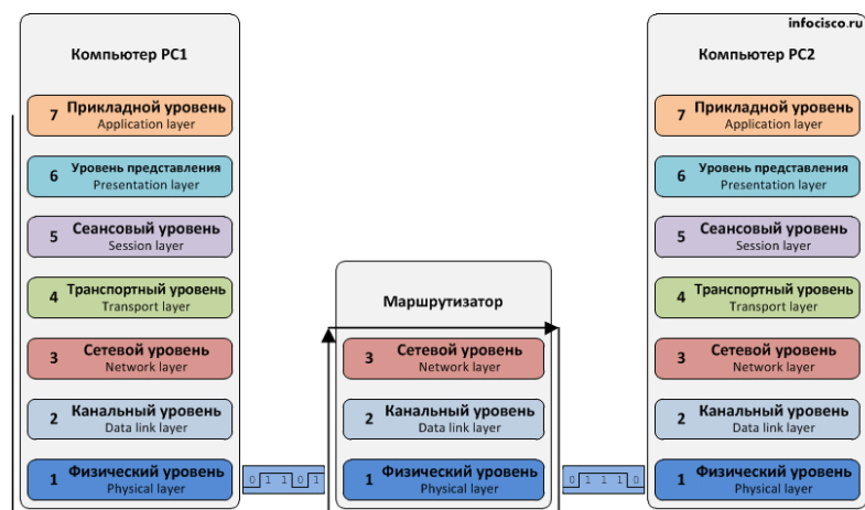
Рисунок 1 – Схема уровней сетевой модели OSI
